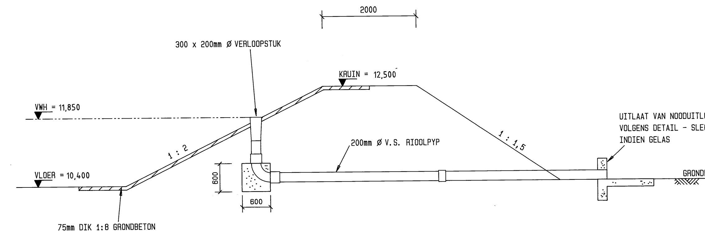
SNIT D - D SNIT DEUR WAL BY NOODUITLOOP 1 : 50
