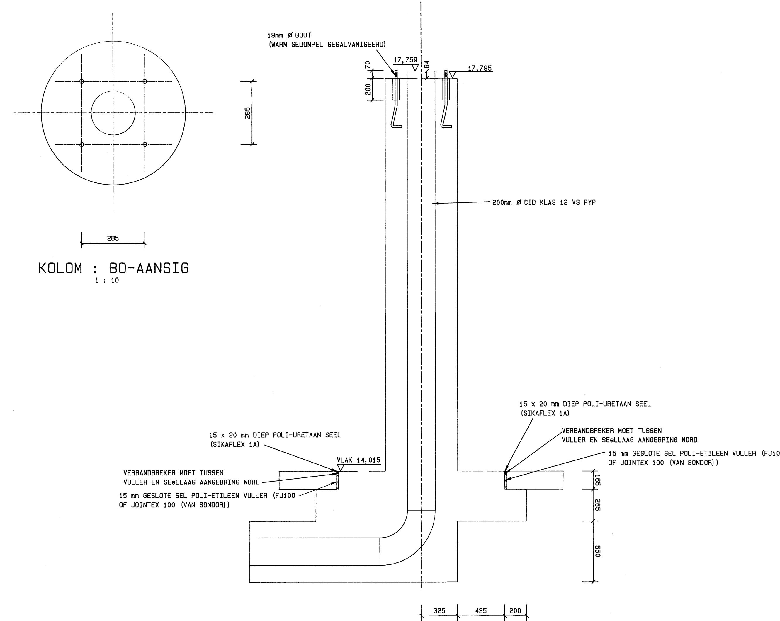
DETAIL VAN MIDDELKOLON SKAAL 1 : 20
