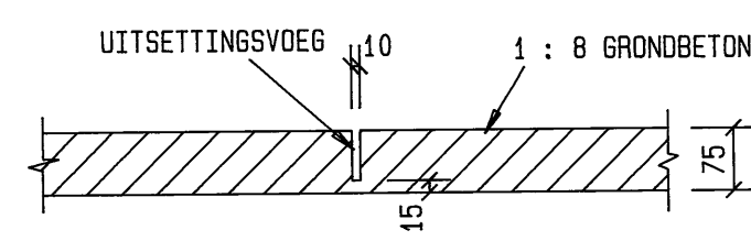
DETAIL VAN UITSETVOEG BY GRONDBETON 1 : 10
