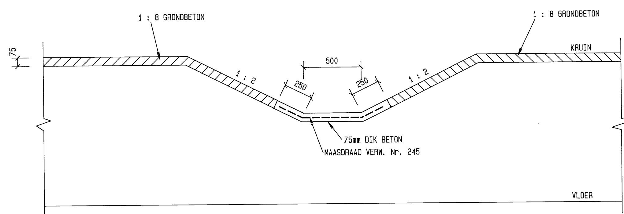
SNIT D1 - D1 1 : 20
