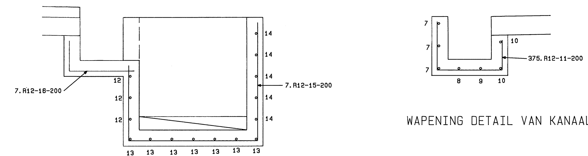
WAPENING DETAIL VAN UITLEATKAS
