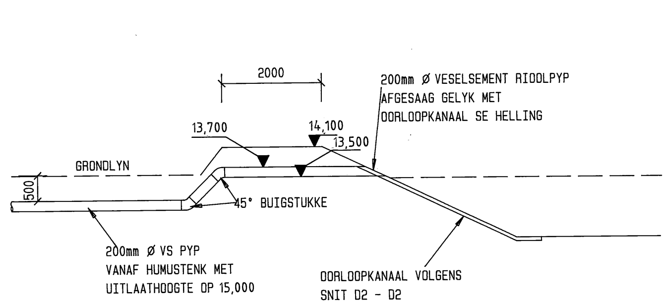
SNIT INLAAT IN VEROUDERINGSDAM N° 1 VANAF HUMUSTENK 1 : 75
