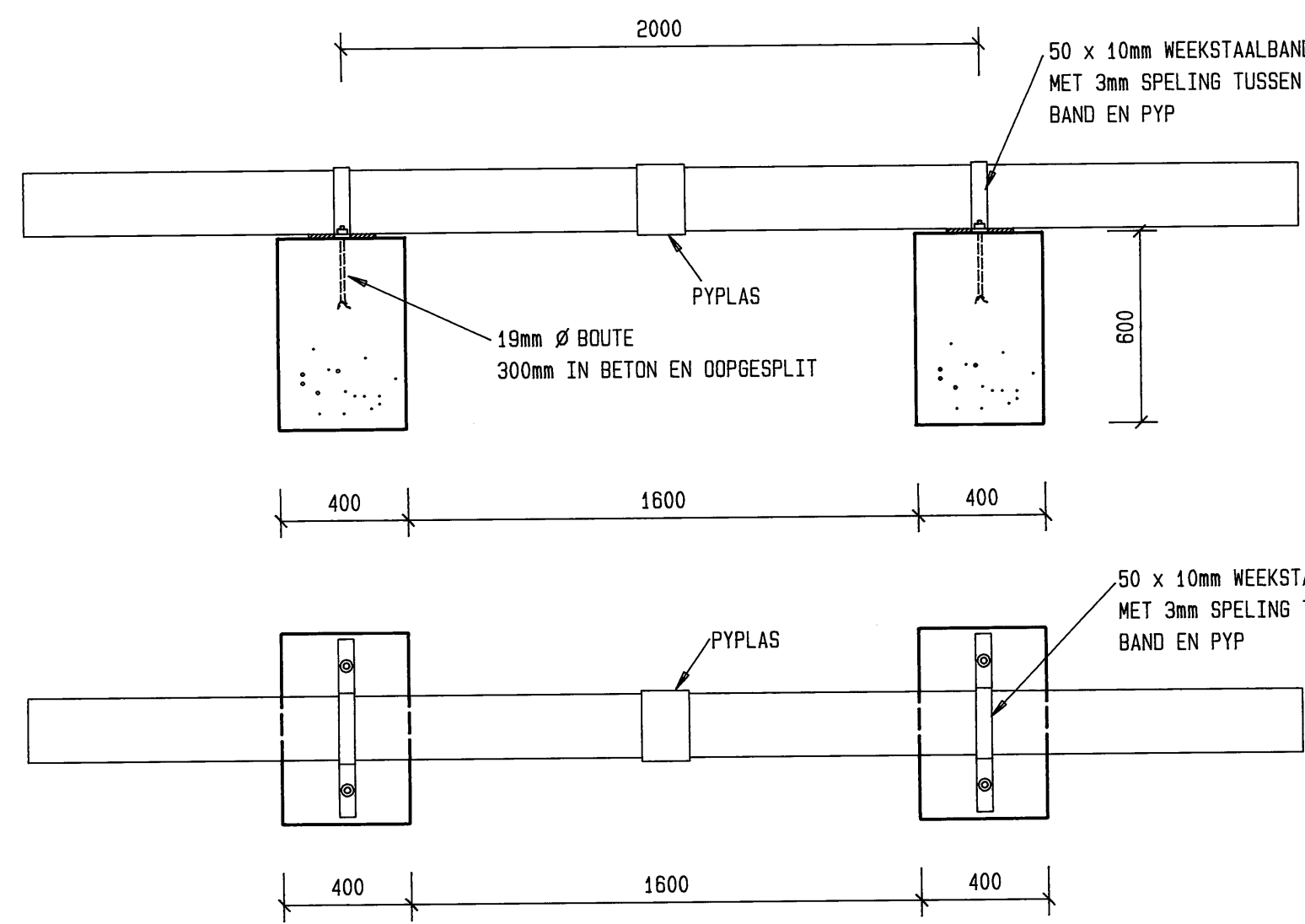
PYP OP BETONBLOKKE 1 : 20
