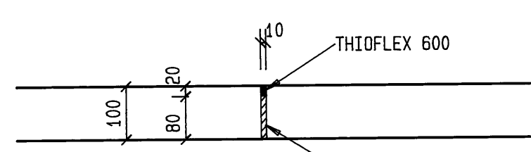
DETAIL VAN UITSETVOEG BY OORLOOP 1 : 10
