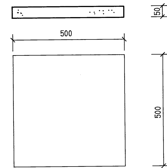
BETON PLAVEISEL 1 : 10
