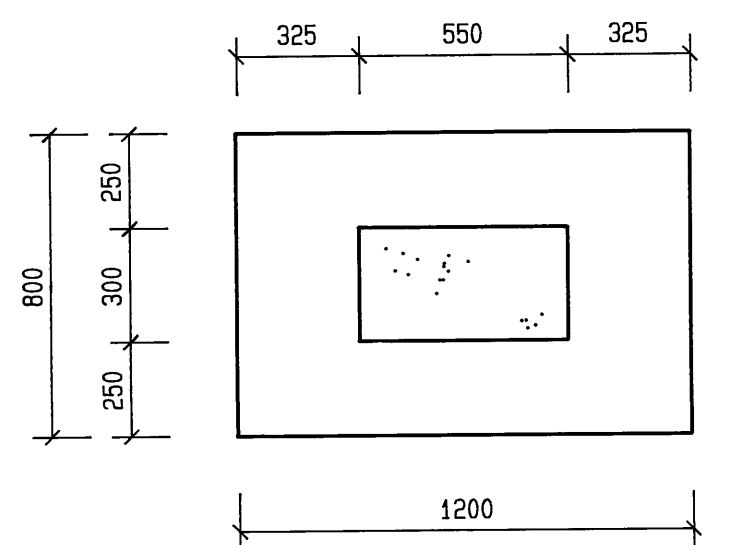
PLAN VAN BETON PILAAR 1 : 20
