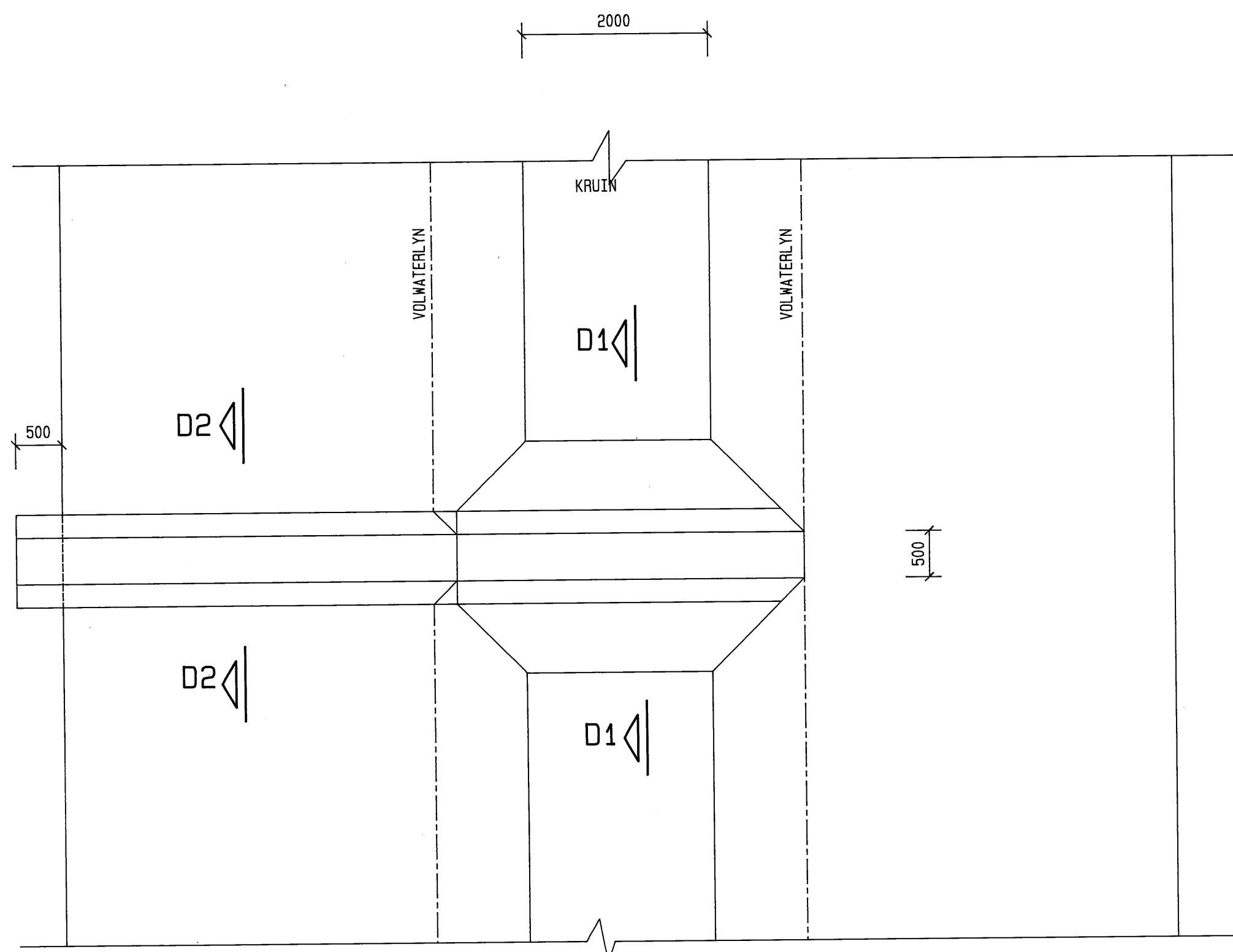
DETAIL VAN UITSETVOEG BY OORLOOP 1 : 10
