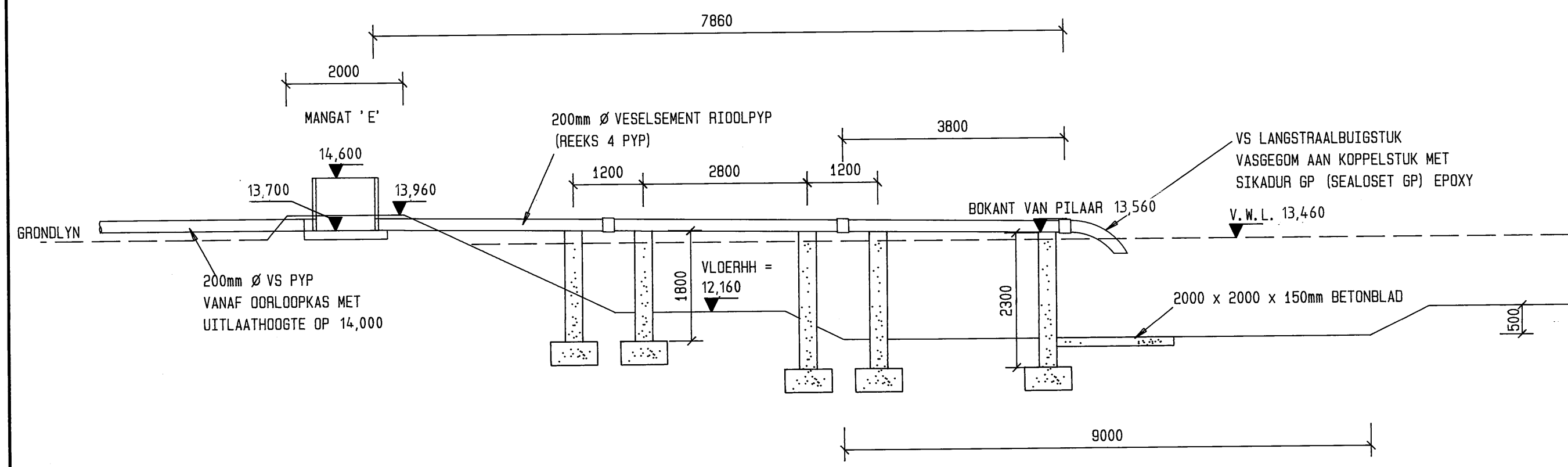
SNIT INLAAT IN SPITSVLOEISTOORAM VANAF OORLOOPKAS 1 : 75
