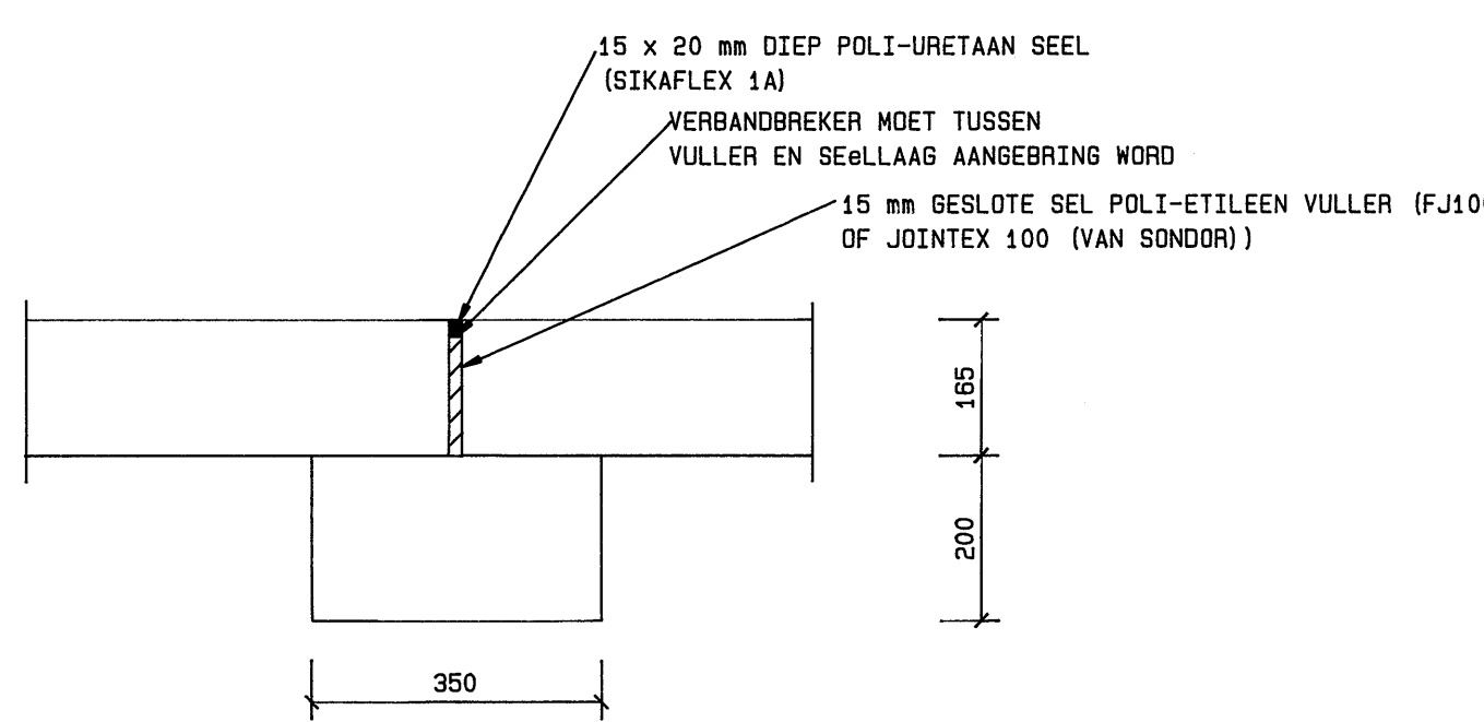
SNIT CC SKAAL 1 : 10
