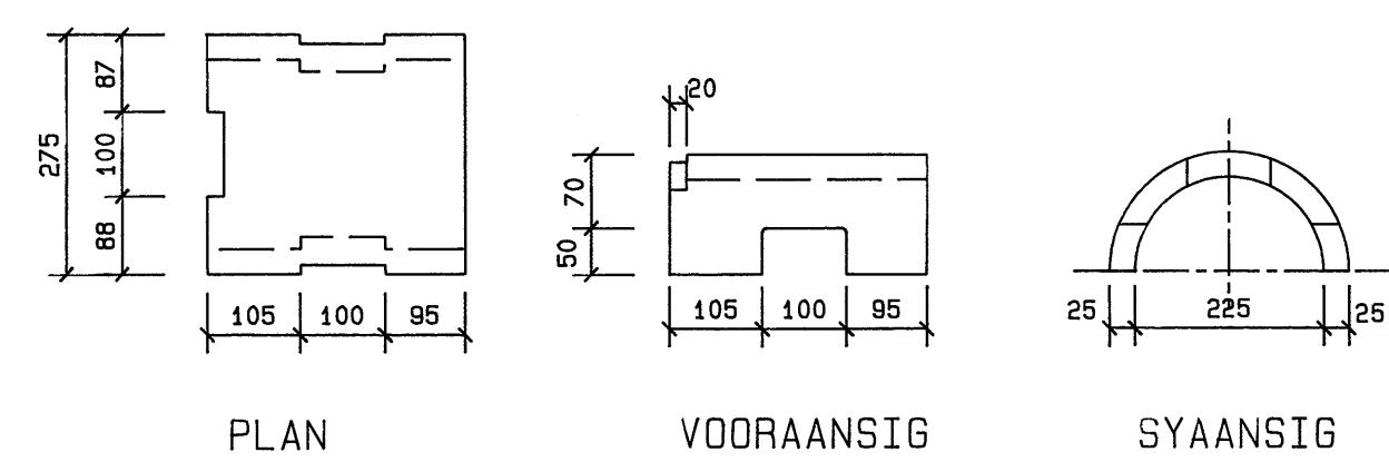
DETAIL VAN BELUGTINGSTEEL SKAAL 1 : 10
