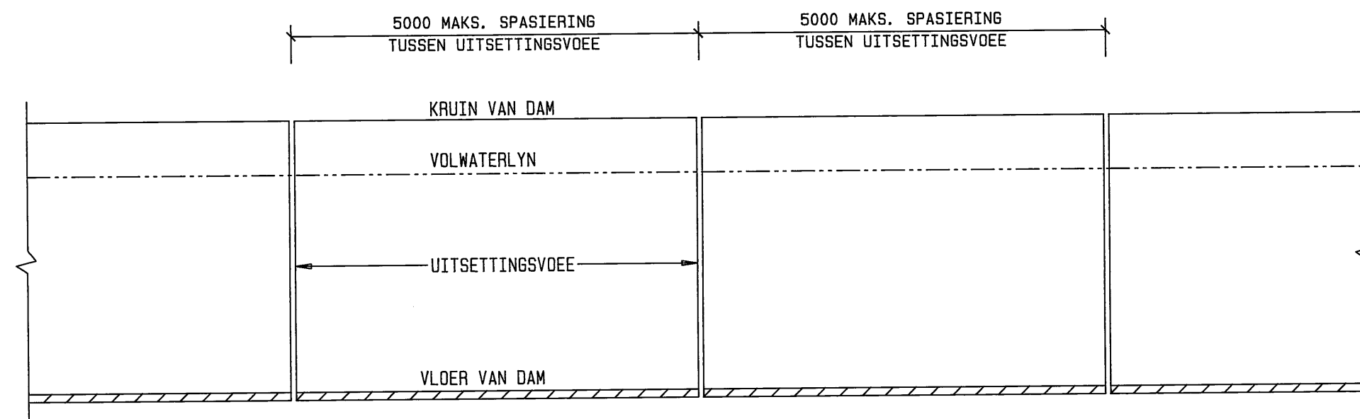
PLAN - SPASIERING VAN UITSETTINGSVOEE N.V.S.
