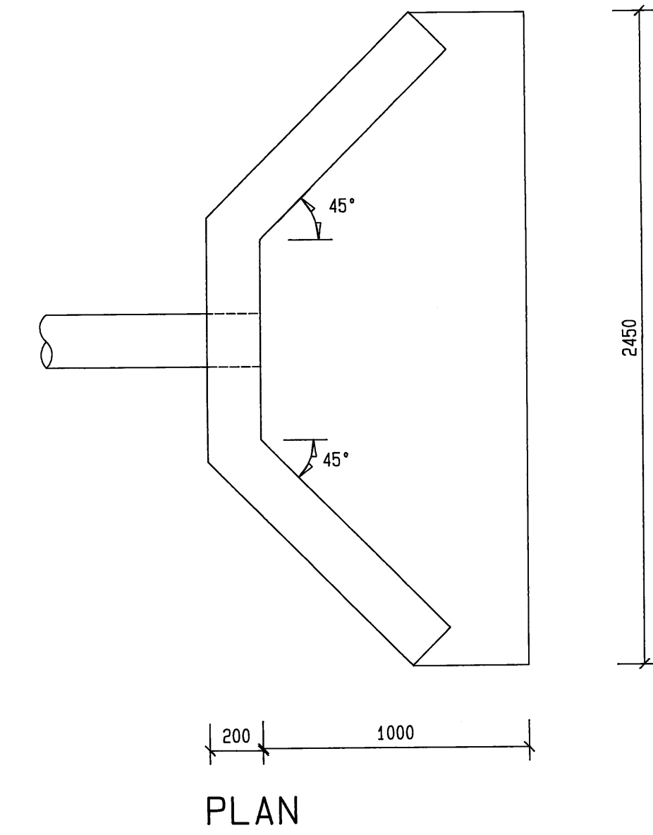
DETAIL VAN UITLOOP VIR NOODUITLOOP 1 : 20
