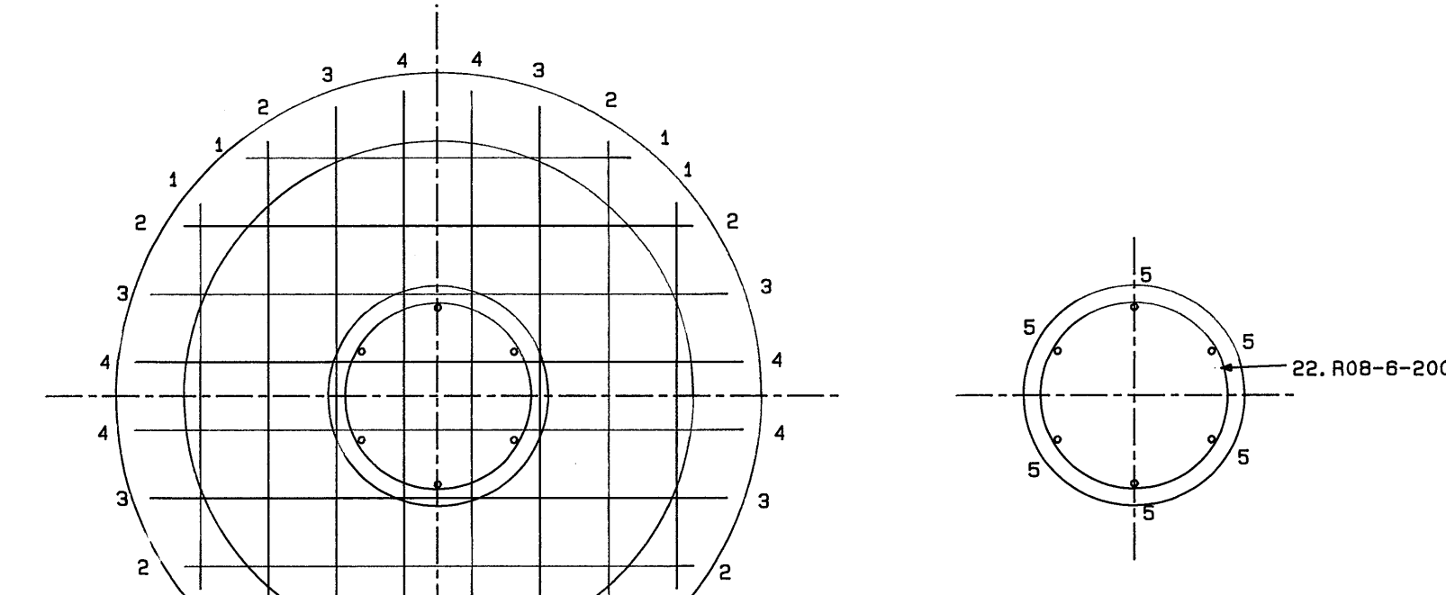
WAPENING UITLEG VAN SENTERKOLON
