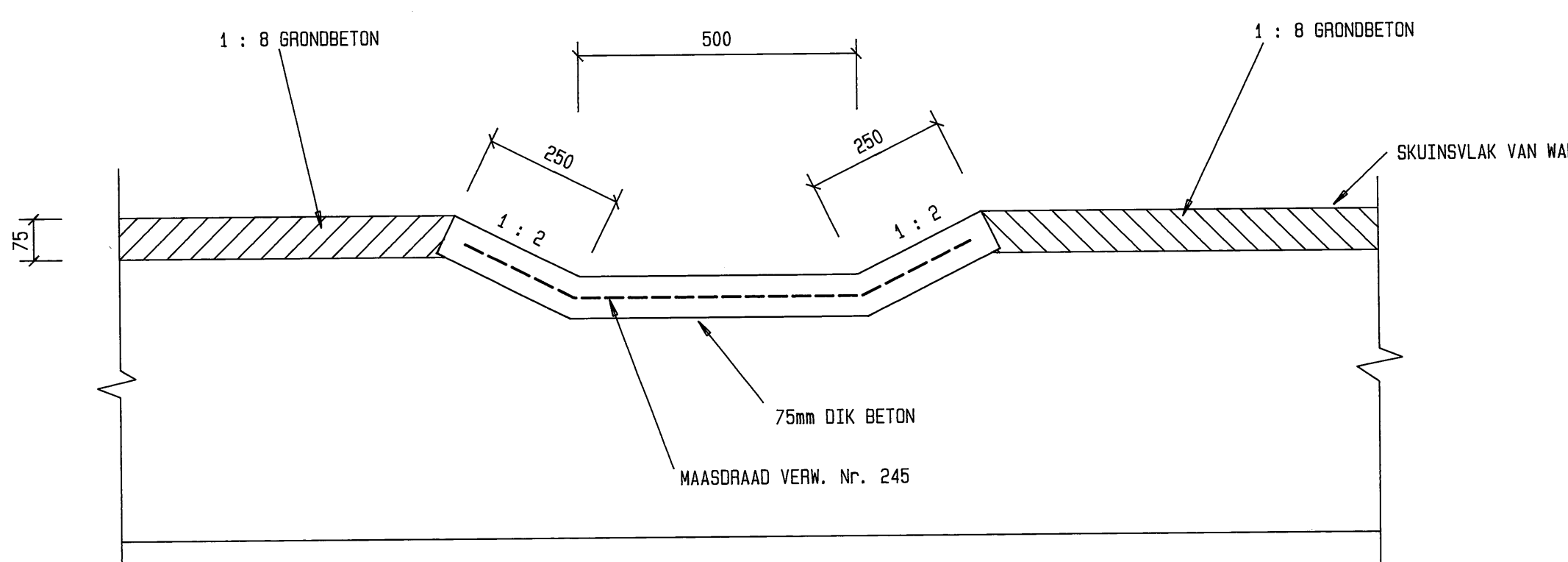
SNIT D2 - D2 1 : 10
