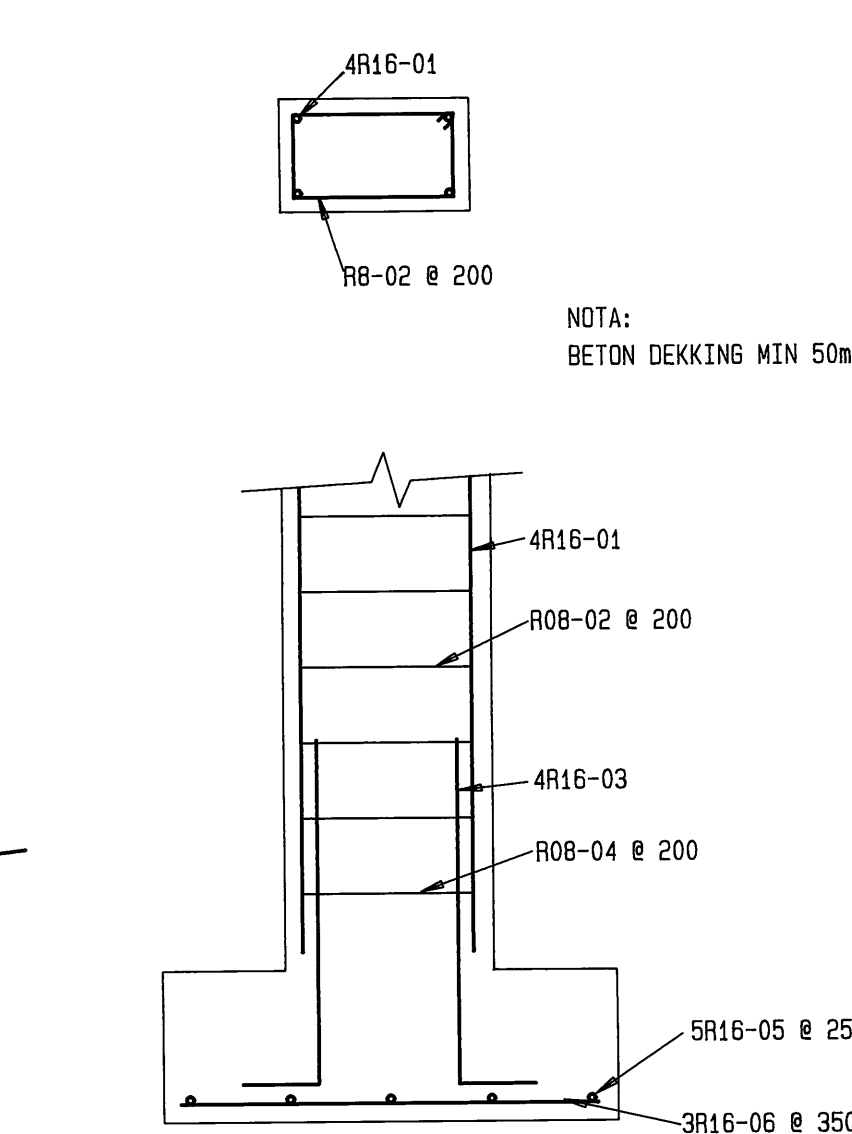
BETON BEWAPENING DETAIL 1 : 20
