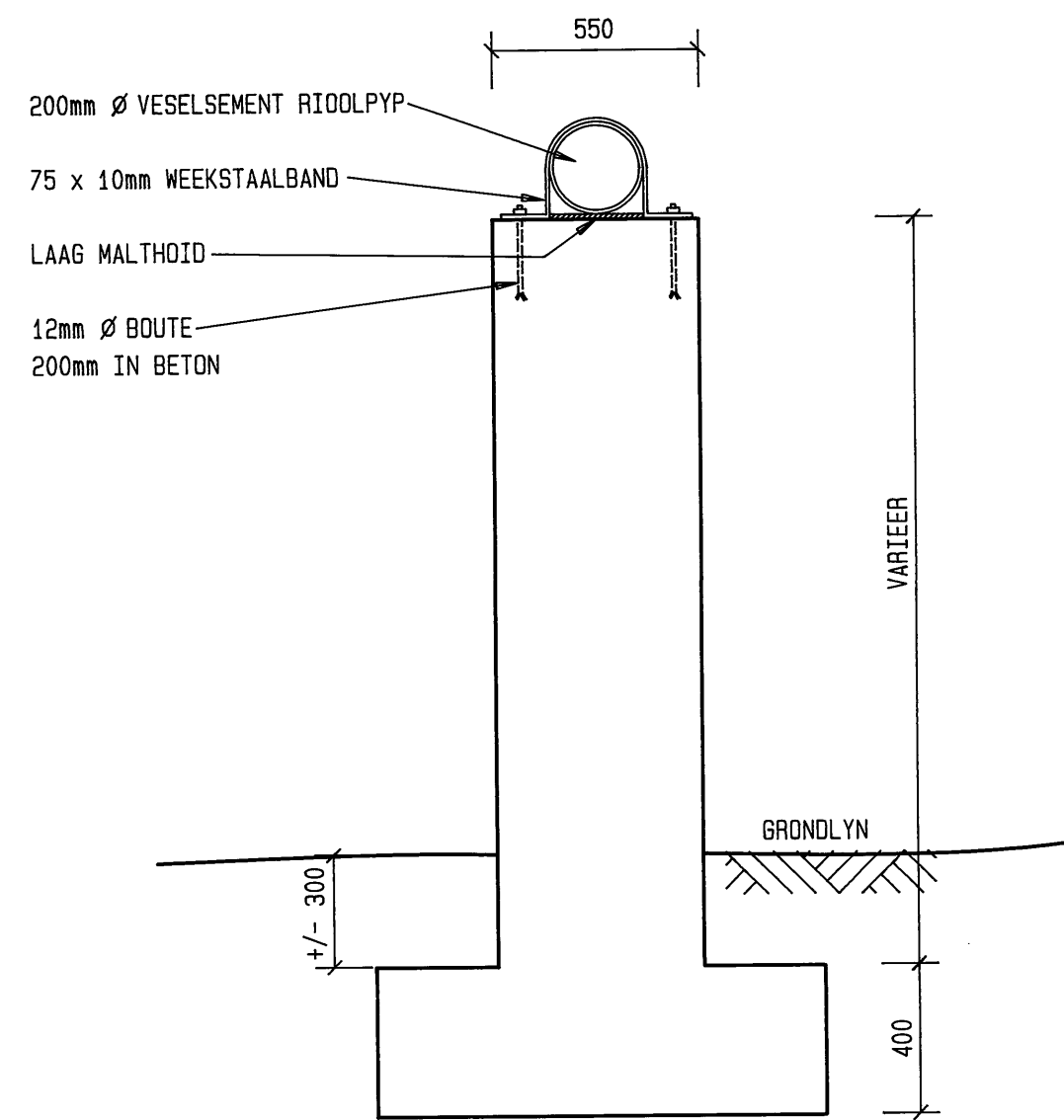
BETON PILAAR 1 : 20
