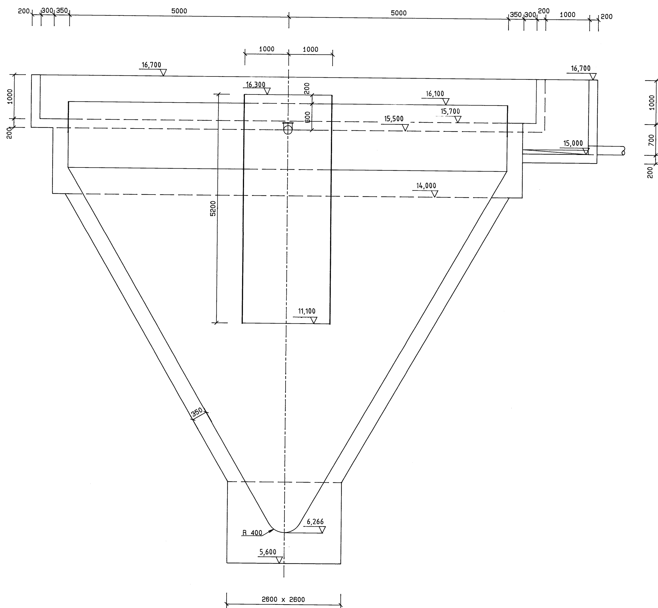
SNIT BB
