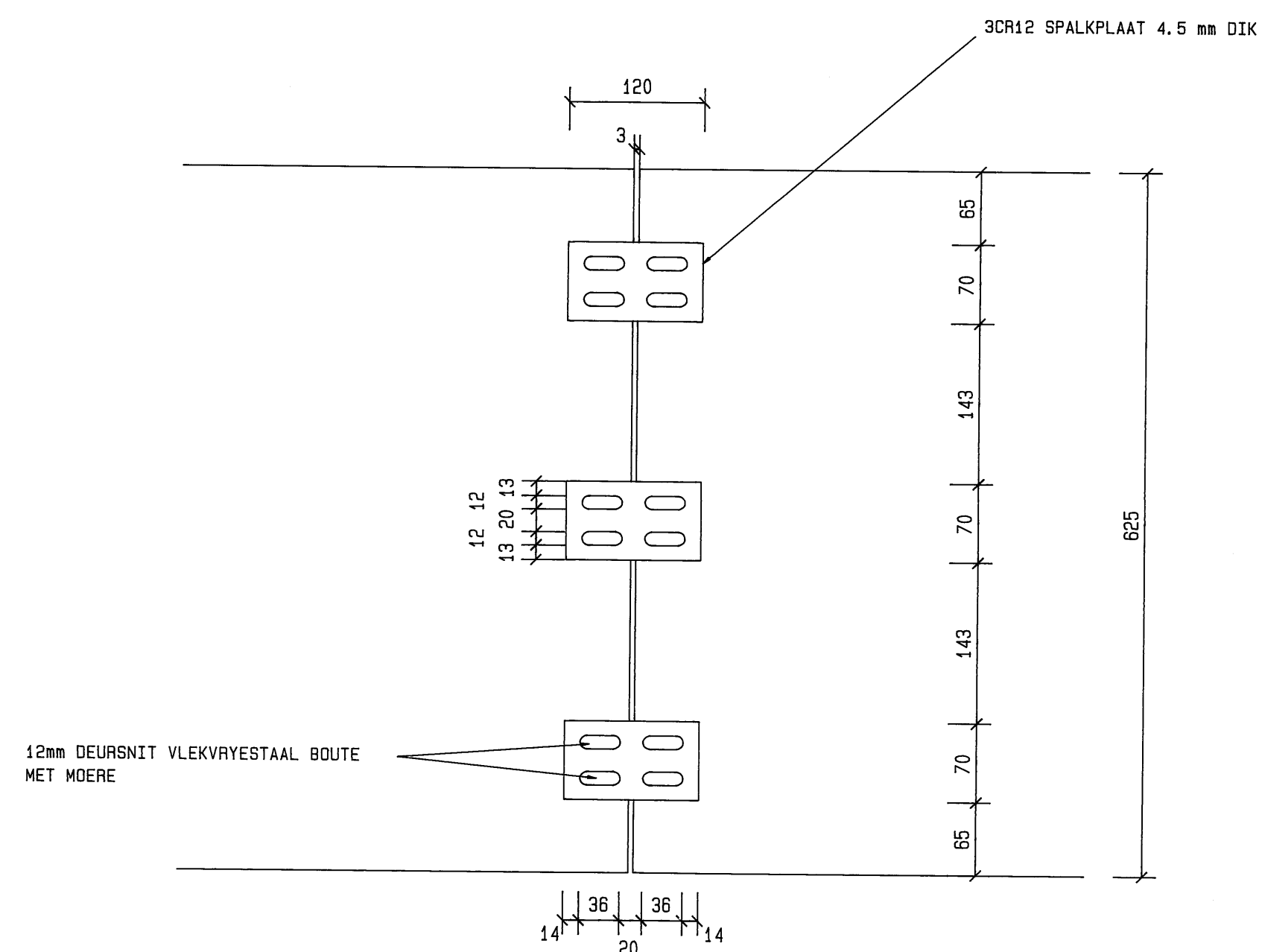
DETAIL 2 : SPALKPLATE
