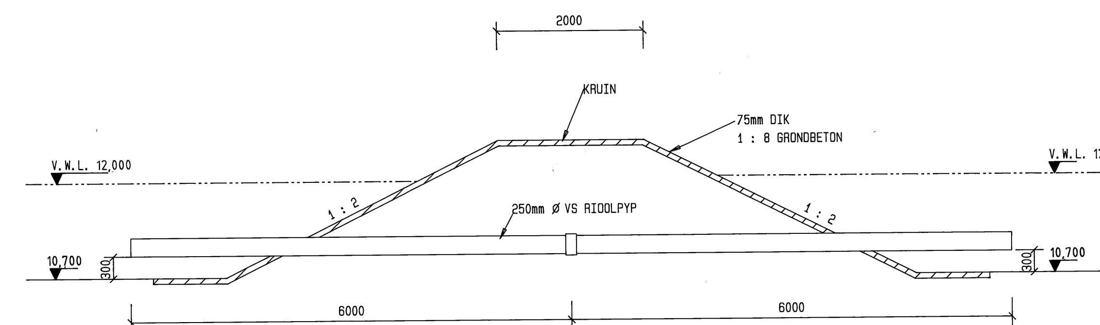
SNIT C - C SNIT VAN OORLOOP TUSSEN VEROUDERINGSDAMME 2 & 3 1 : 50
