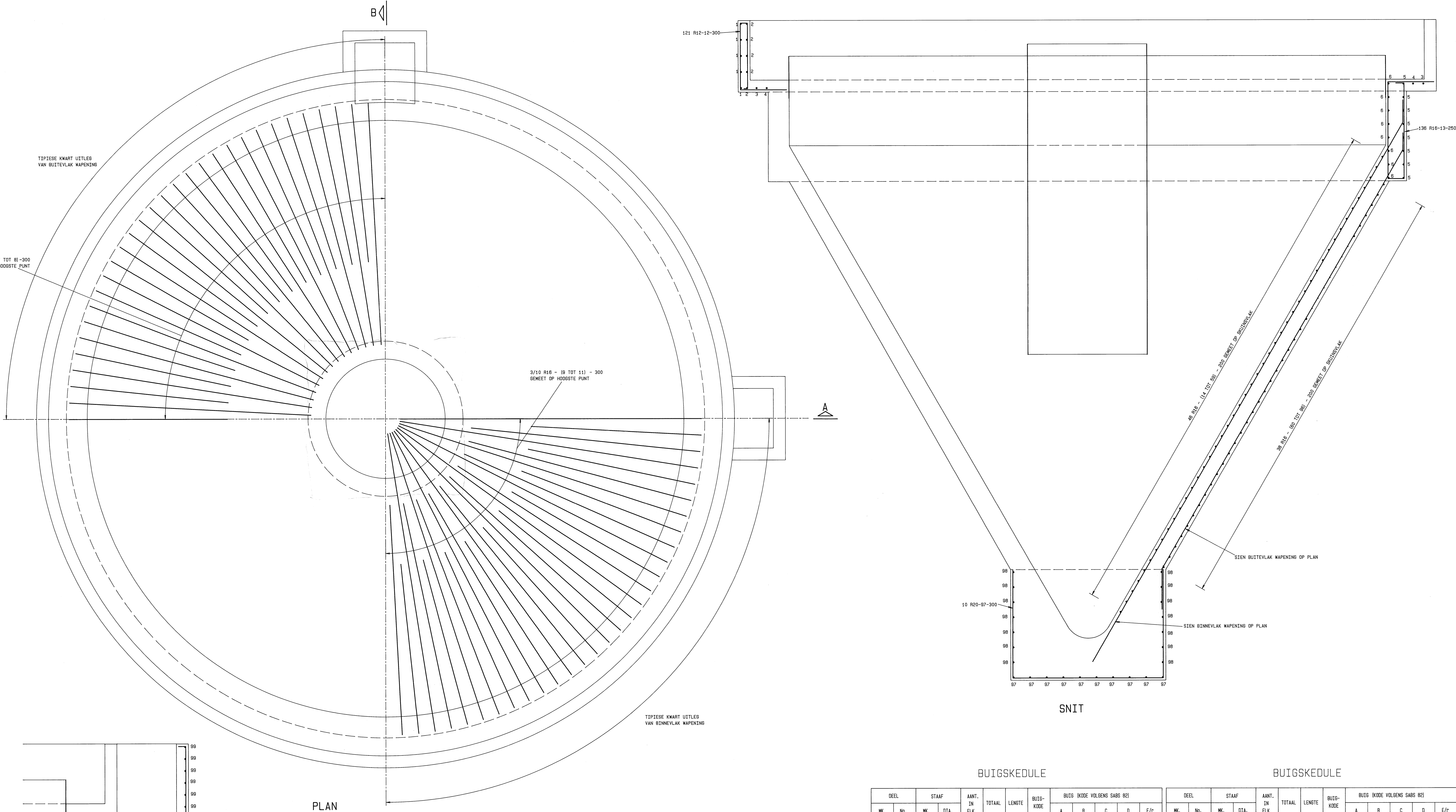
BUIGSKEDULE
